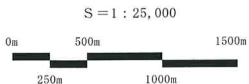
図 3-1-10 土壌図
