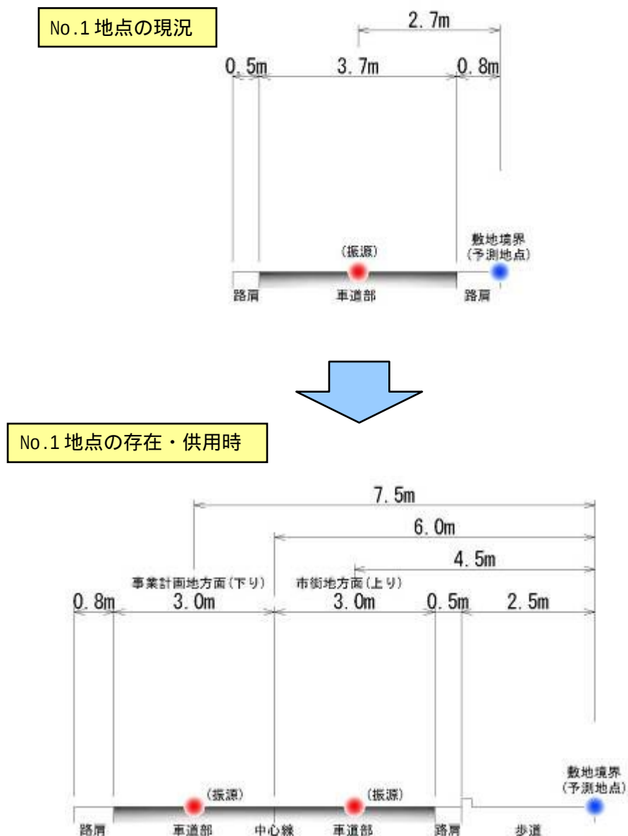
図 7-3-16 予測地点（現況及び存在・供用時の道路構造 No.1）
