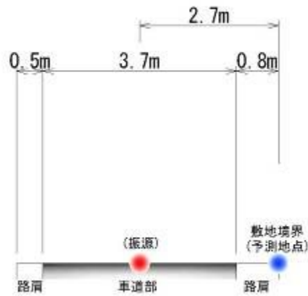
断面図(S=1/100)
