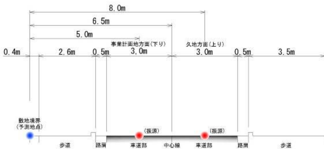
断面図(S=1/100)
