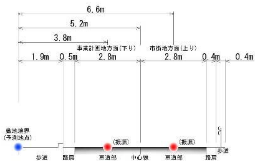
断面図(S=1/100)
