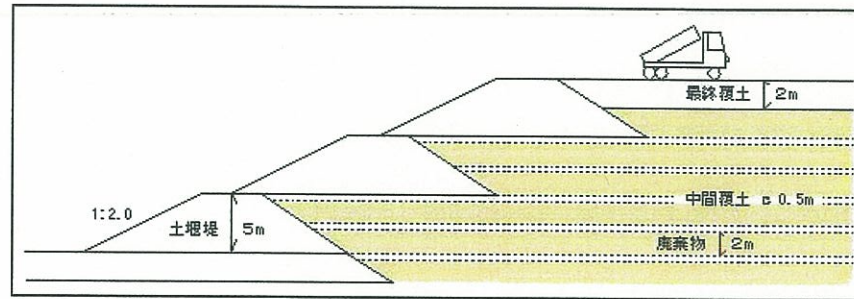
図 2-3.9 サンドイッチ工法
