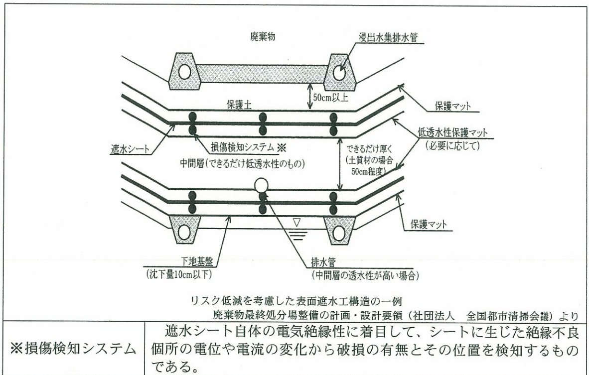
図 2-3.6 遮水工概要図
