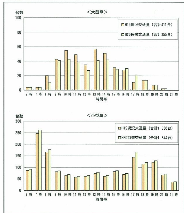
図7-2.12 (2) St. 2 : 県道269号線の将来交通量
