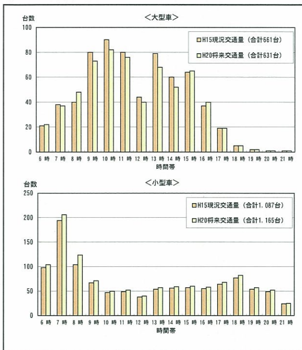
図7-2. 12 (3) St. 3 : 県道177号線の将来交通量
