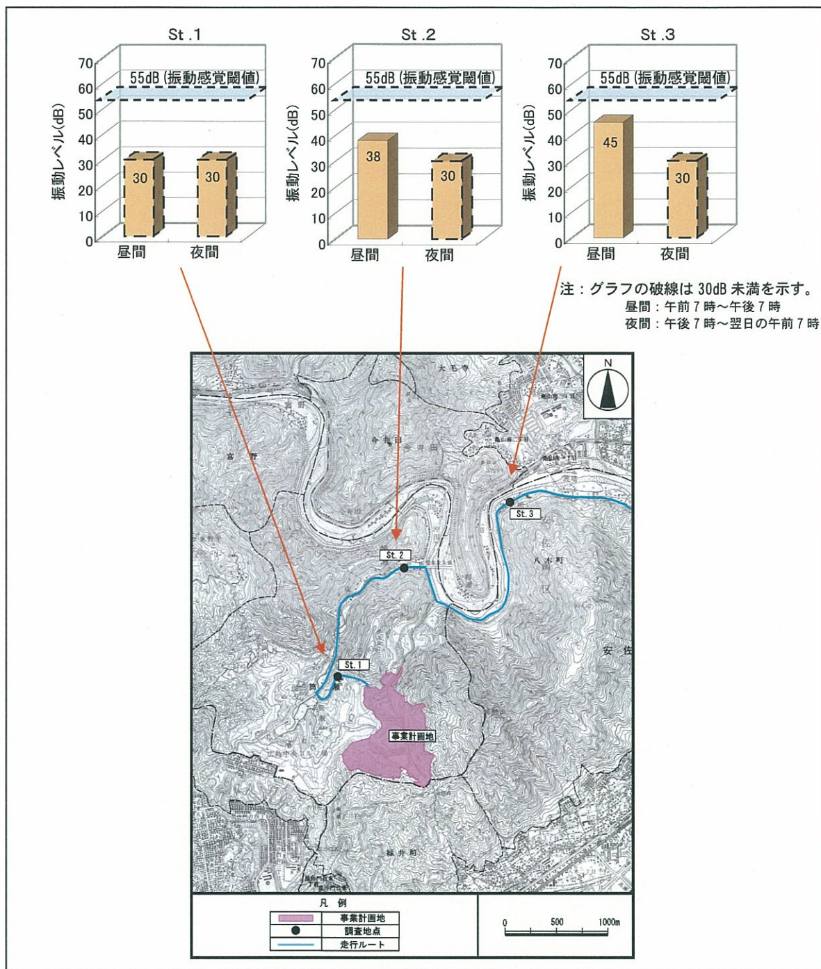
図 7-3.3 道路交通振動調査結果
