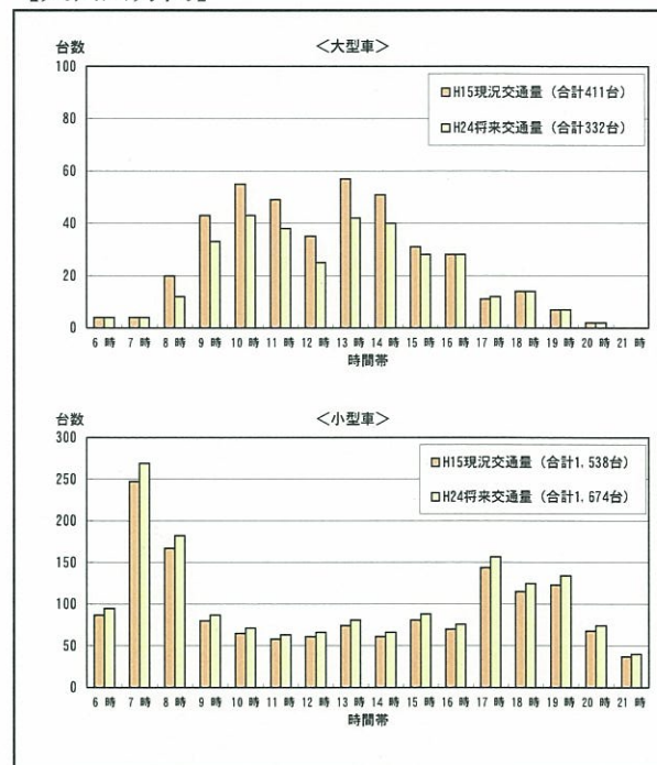
図7-2.23 (2) St. 2 : 県道269号線の将来交通量
