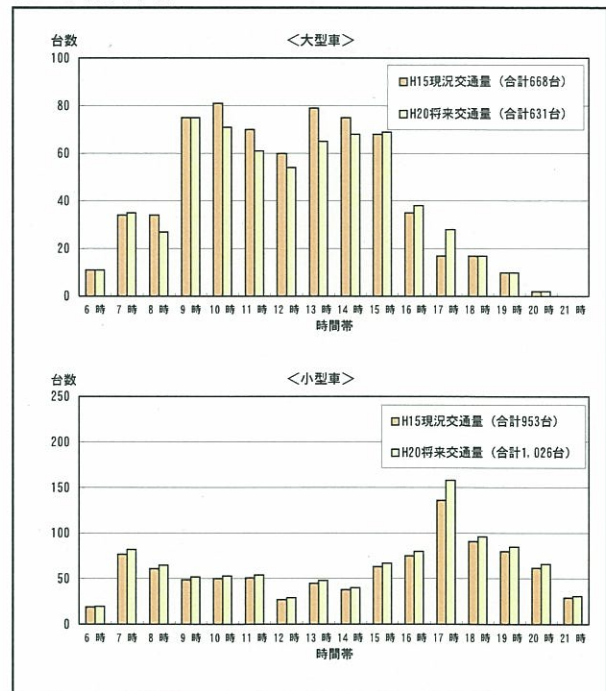
図7-2. 12 (3) St. 3 : 県道177号線の将来交通量
