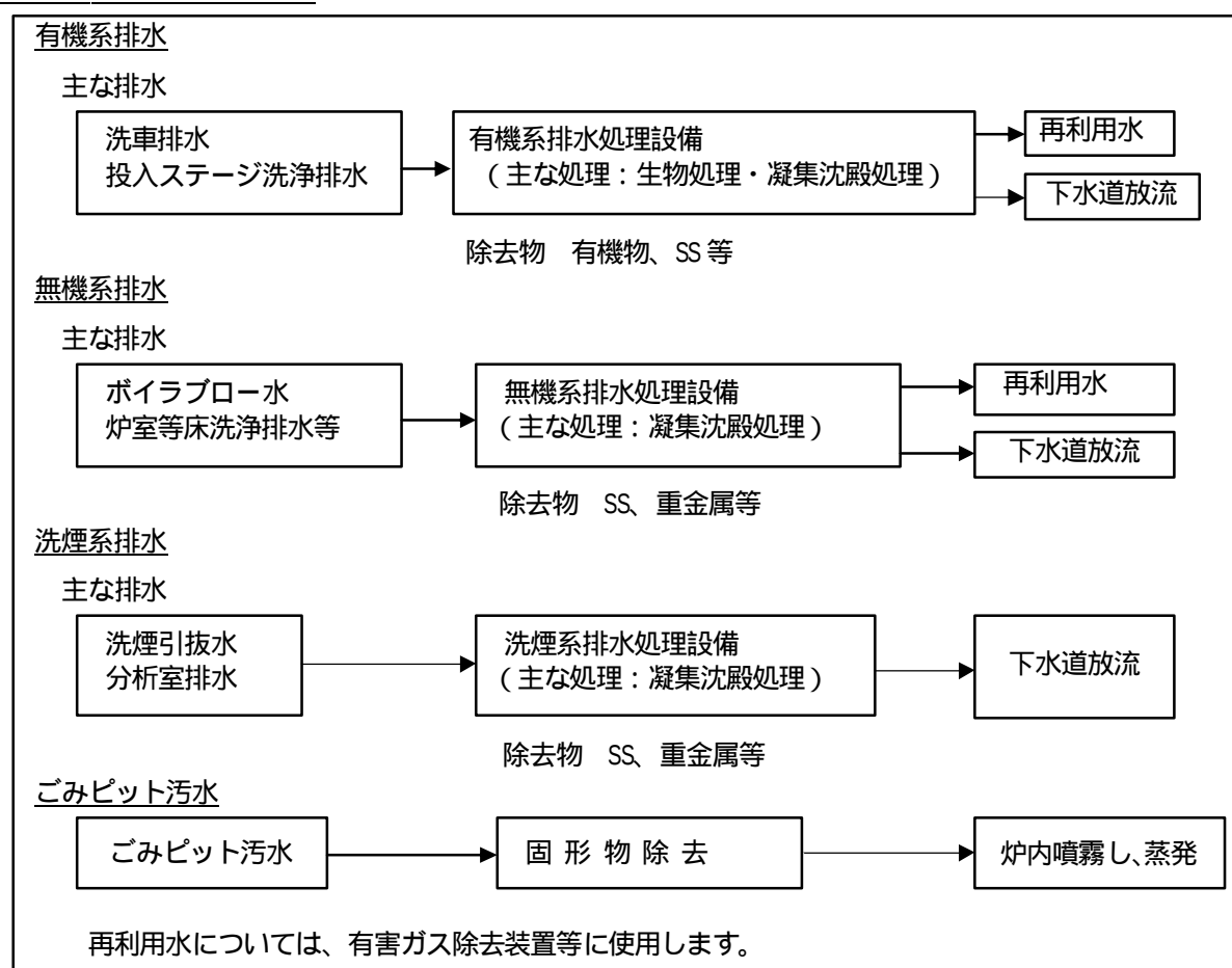
図 -12-1 排水処理フロー
