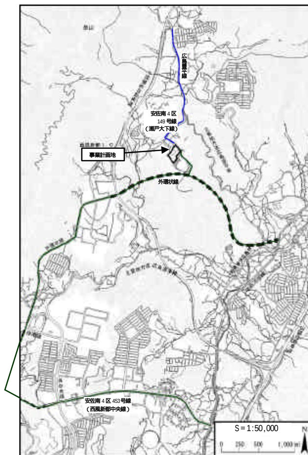
図 -13-1 ごみ収集車搬入ルート（外環状線開通時）
