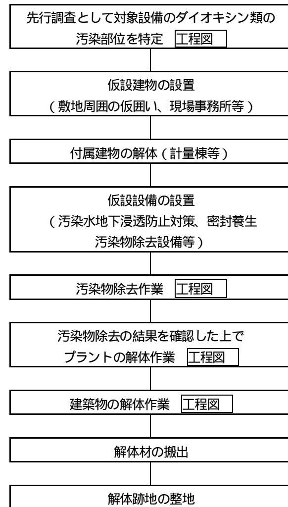
図 -10-1 解体工事の作業工程
