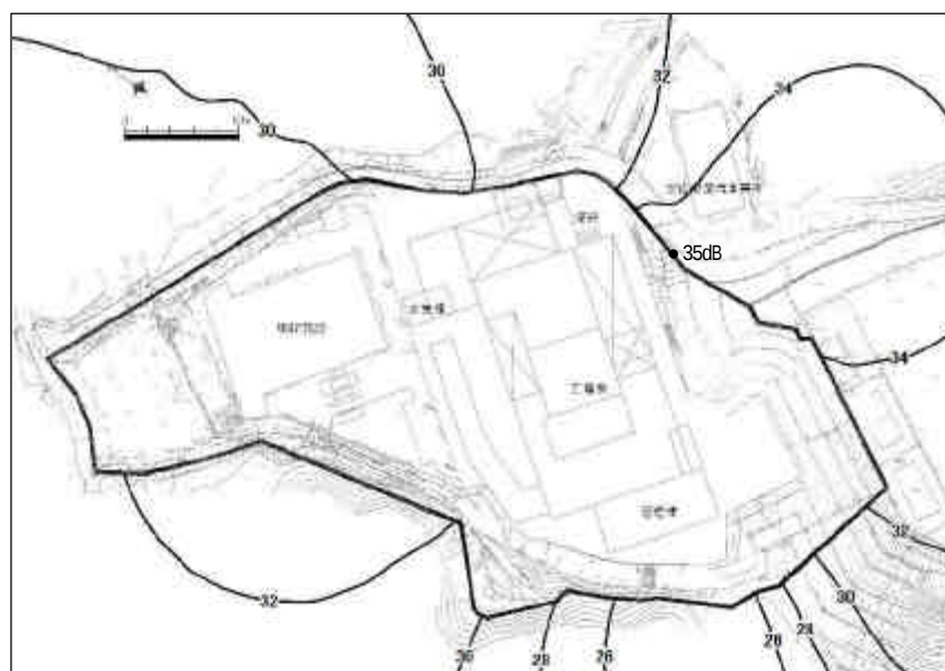
図 -2-6 施設の稼働時に発生する騒音レベルの寄与予測結果（スラグクレーン停止時（朝・夕・夜間））
