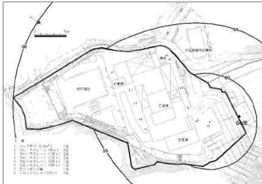
図 -3-3 予測結果 (建築工事)
