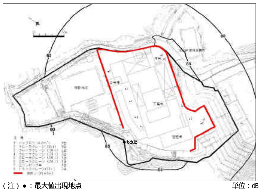
図 -2-4 予測結果（建築工事）
