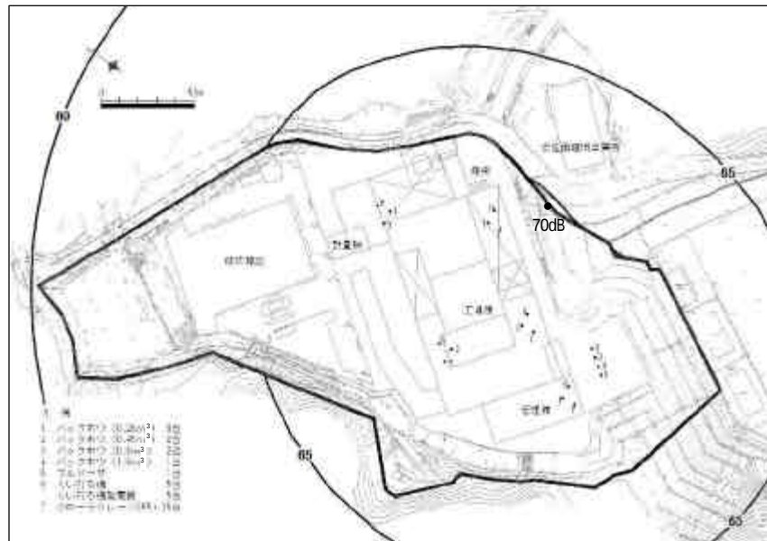
図 -3-2 予測結果 (基礎工事)
