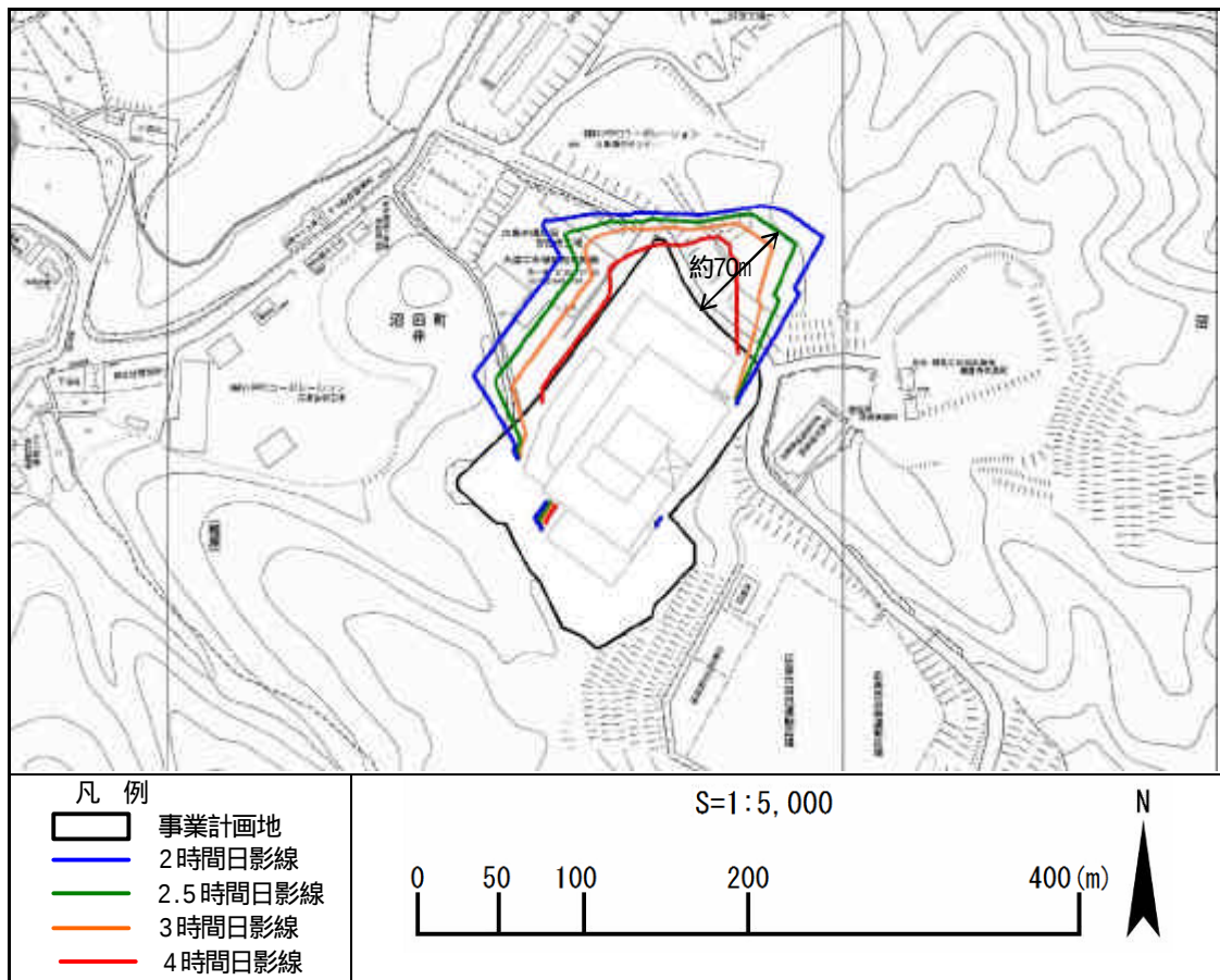
図 -7-1 等時間日影線図
