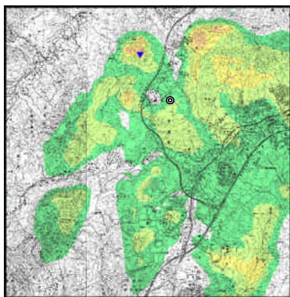
図 -1-2 寄与濃度（年平均値）分布図（施設の稼働・二酸化硫黄）
