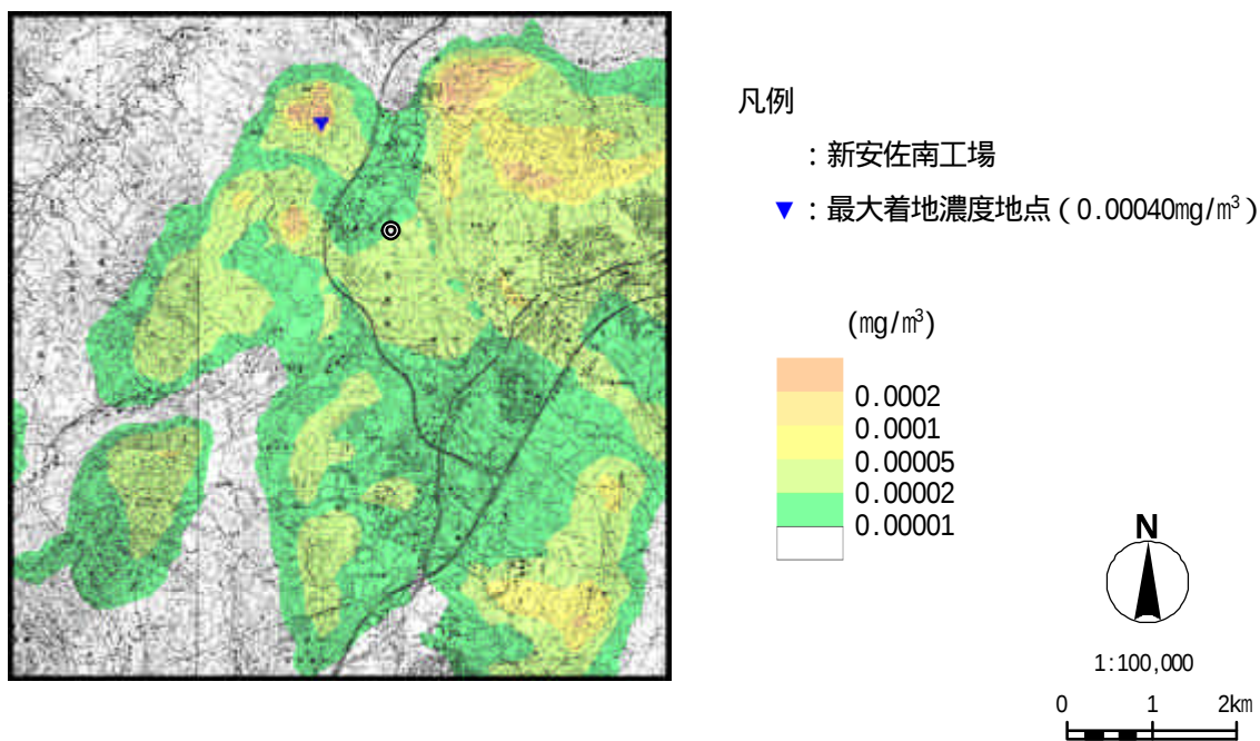
図 -1-4 寄与濃度（年平均値）分布図（施設の稼働・浮遊粒子状物質）
