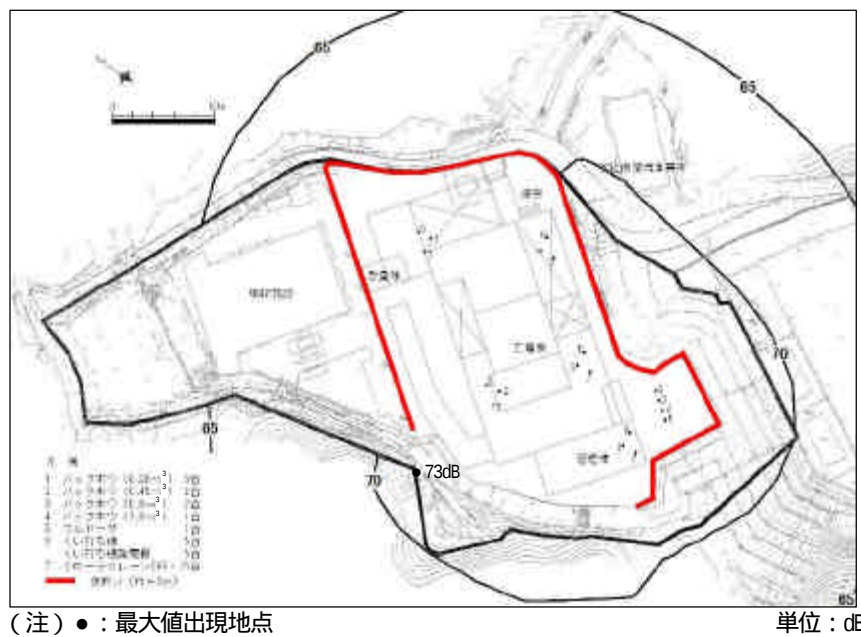
図 -2-3 予測結果（基礎工事）
