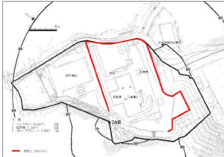
図 -2-2 予測結果（現工場解体工事）
