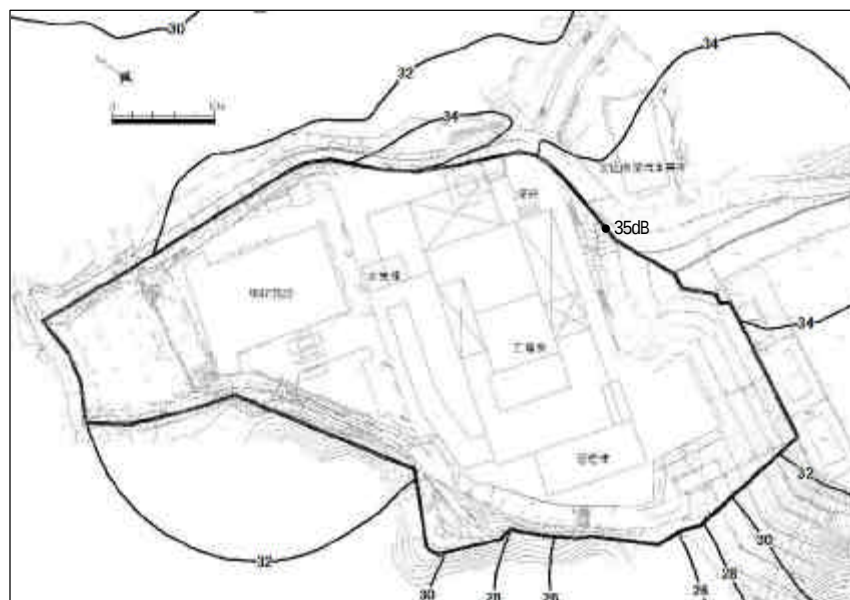
図 -2-5 施設稼働時に発生する騒音レベルの寄与予測結果（全機器稼働時（昼間））
