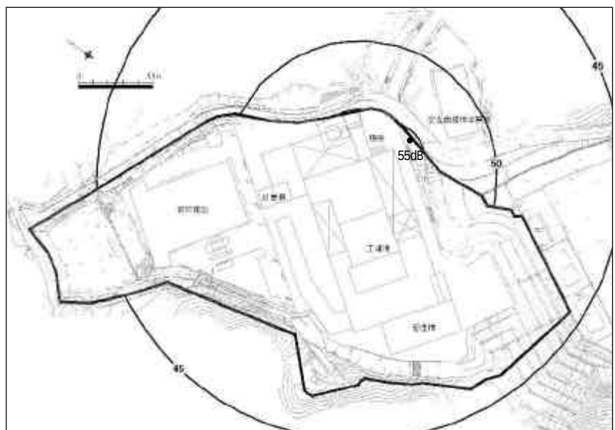
図 -3-4 予測結果（施設の稼働）
