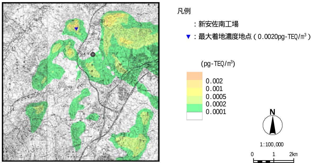
図 -1-6 寄与濃度（年平均値）分布図（施設の稼働・ダイオキシン類）
