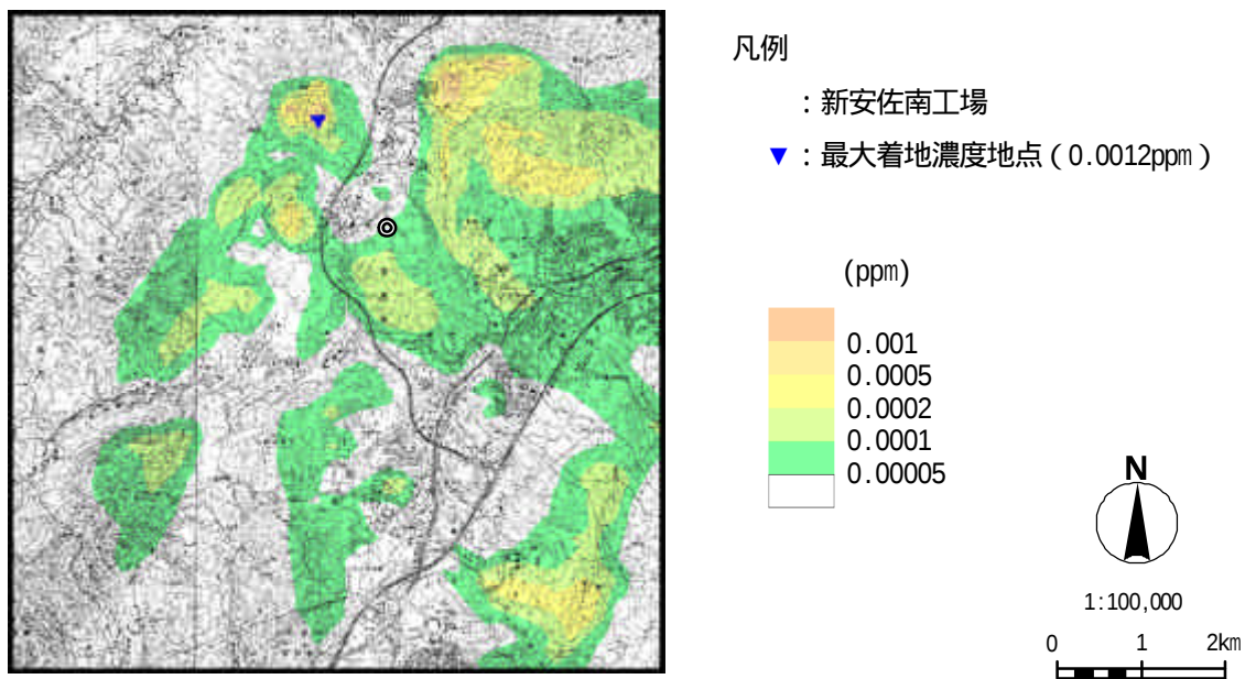
図 -1-5 寄与濃度（年平均値）分布図（施設の稼働・塩化水素）
