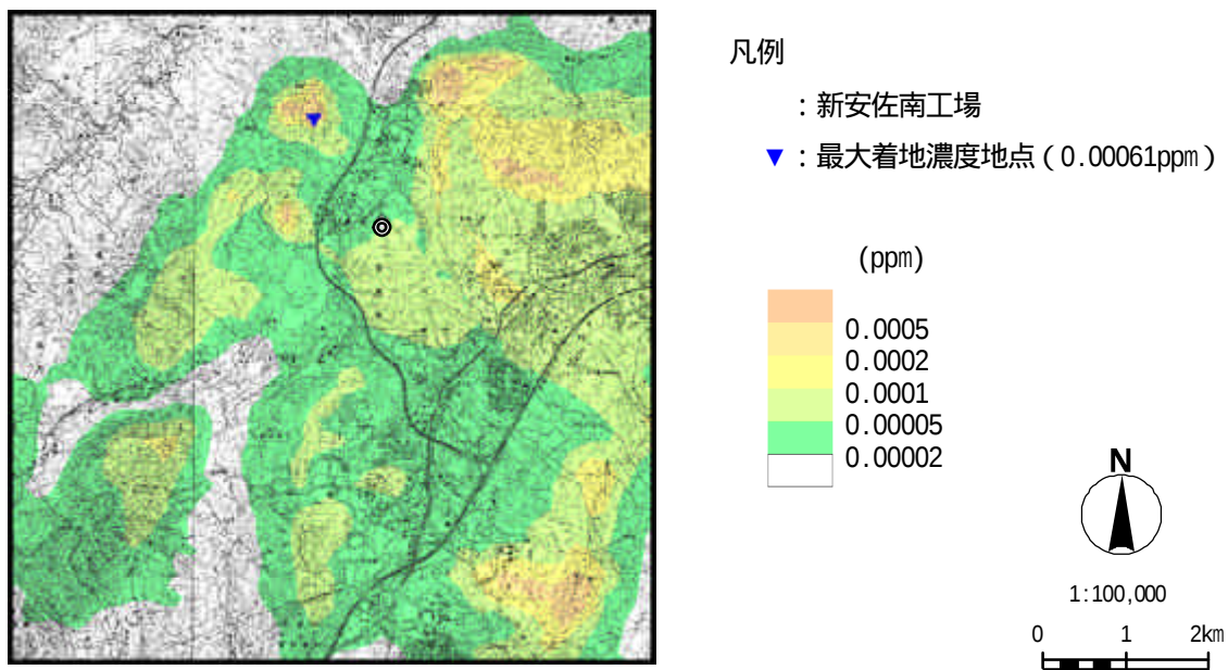
図 -1-3 寄与濃度（年平均値）分布図（施設の稼働・二酸化窒素）
