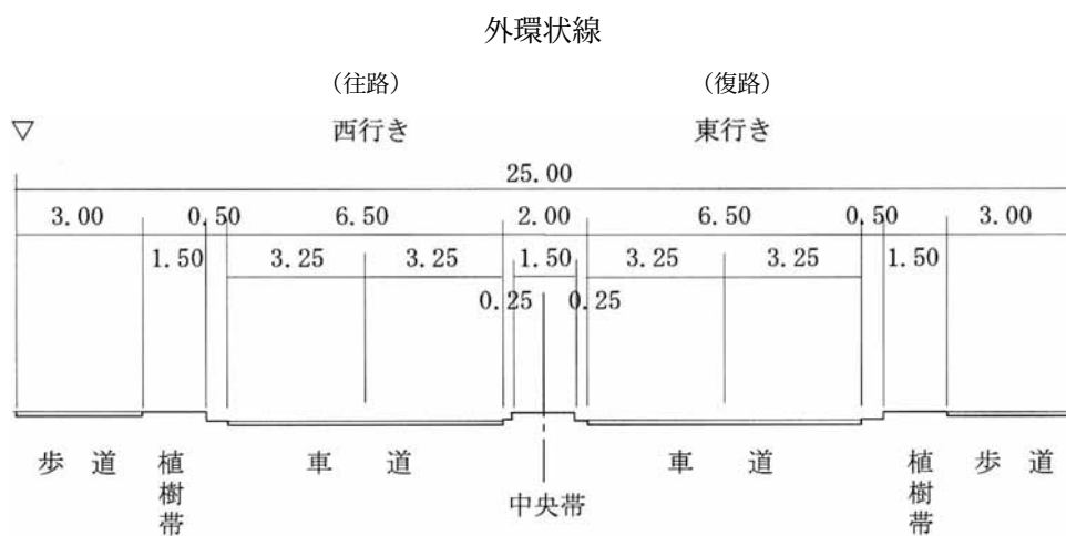
図 7.1.2-11(3) 道路断面図
