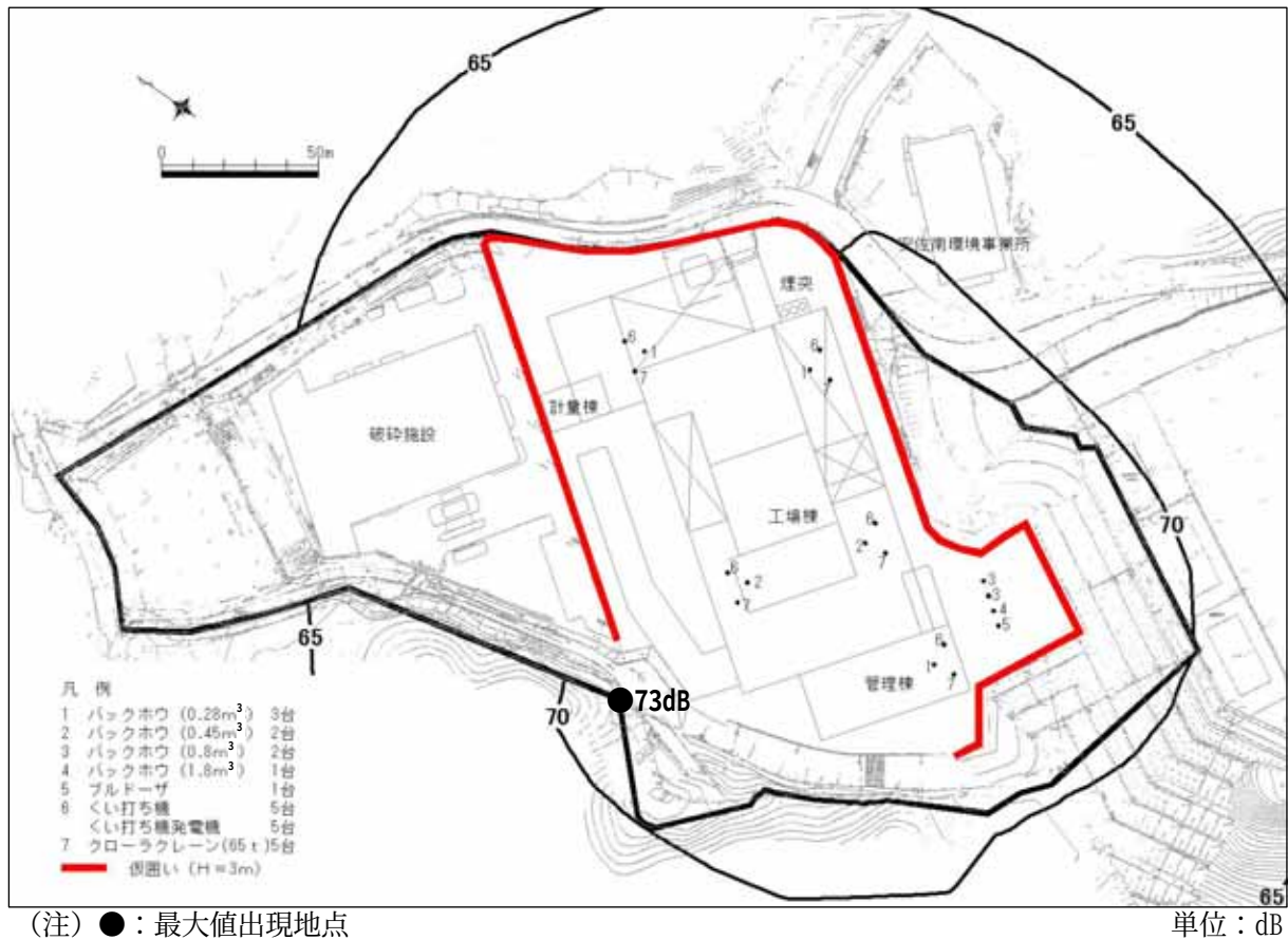
図 7.1.2-13(1) 周辺の騒音レベルの予測結果（基礎工事）
