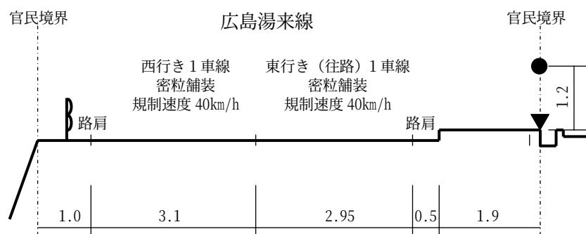
図 7.1.2-11(4) 道路断面図
