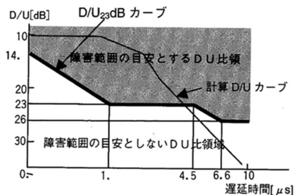
図 7.9.5 障害とする D/U_{23} dB カーブ
