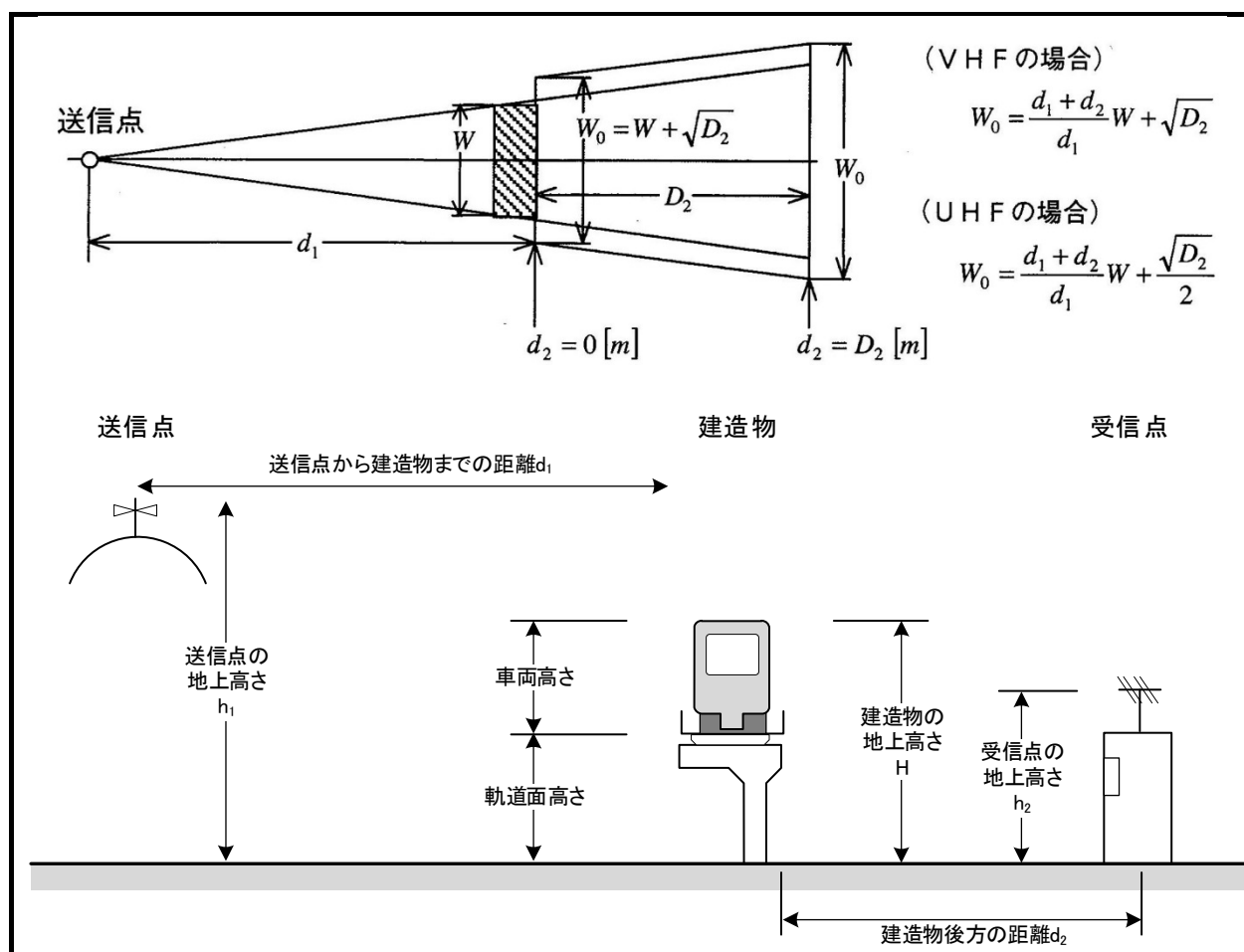
図 7.9.3 遮蔽障害予測の概要
