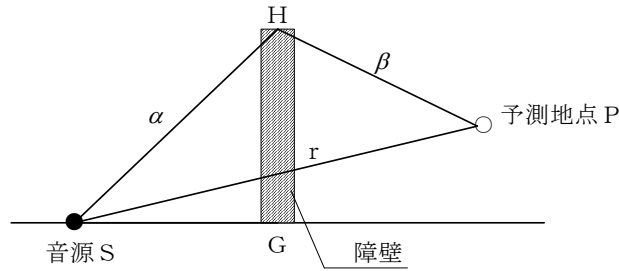
図 7.2.16 音源、予測地点及び障壁の位置関係
