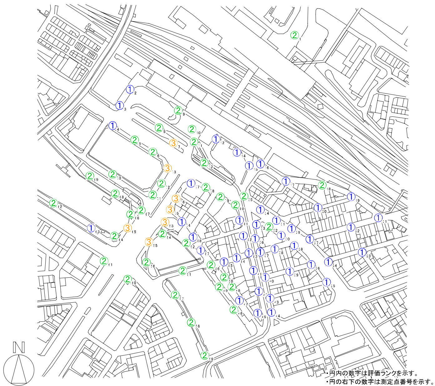
図 7-2-6-5 (2) 風環境評価ランク結果（建設前B）
