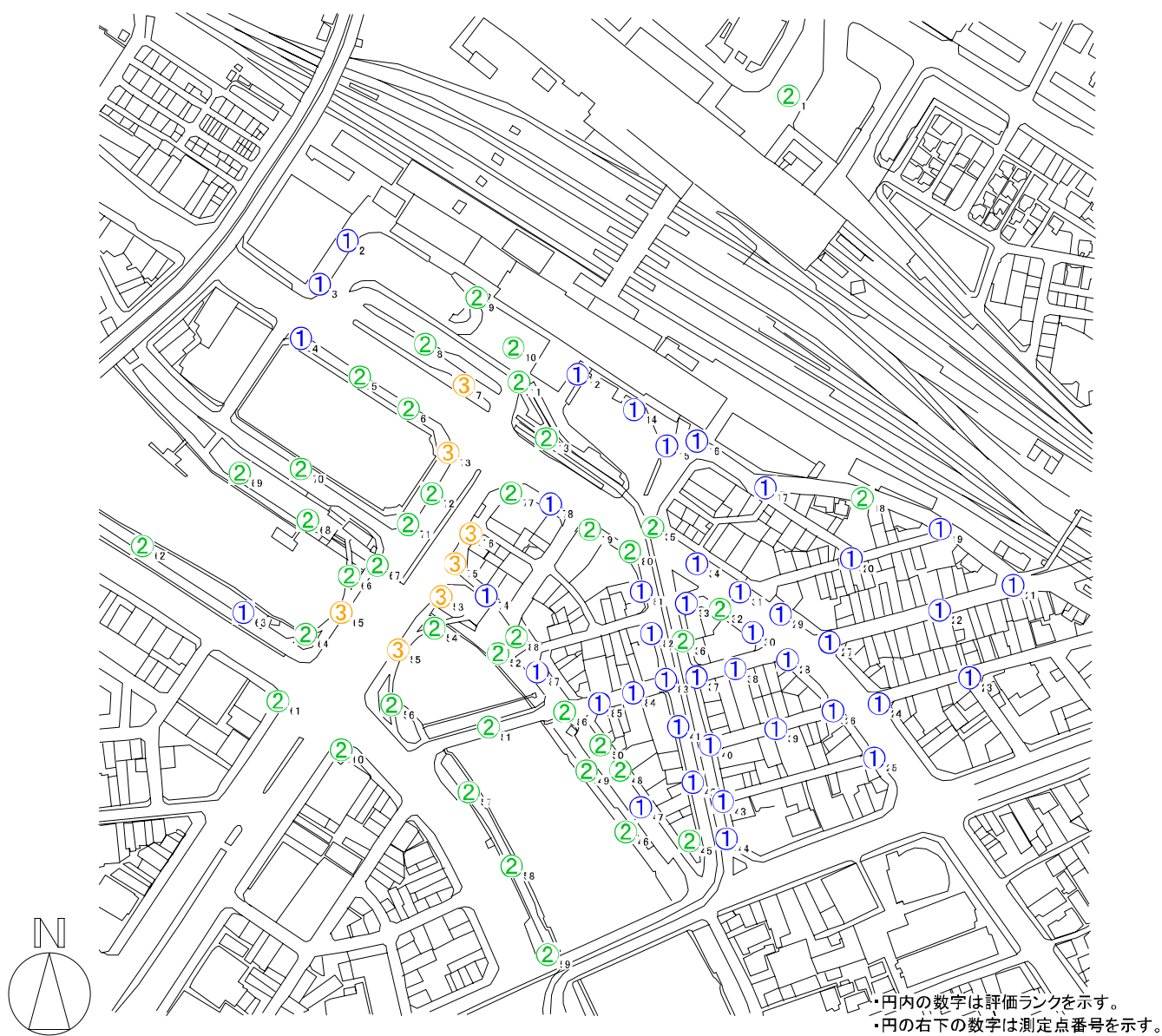
図 7-2-6-5(1) 風環境評価ランク結果 (建設前 A)
