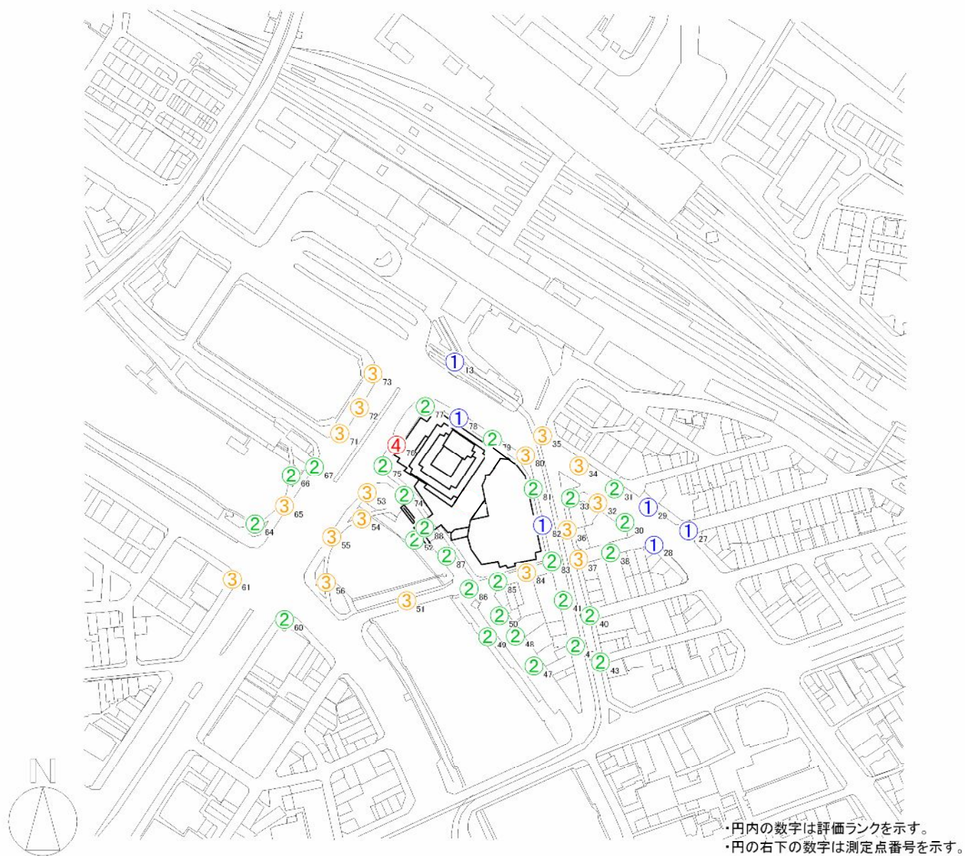
図 7-2-6-6(3) 風環境評価ランク結果（対策考慮）
