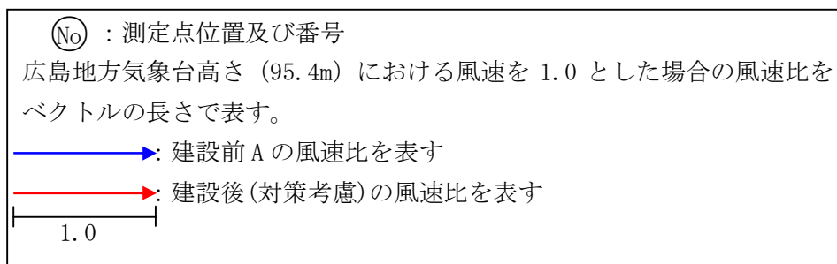
図 7-2-6-7(3) 建設前後の風向・風速比ベクトル図 (建設前 A と建設後 (対策考慮))
