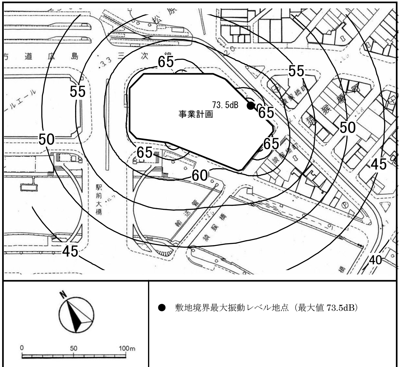
図 7-2-3-4 建設作業振動の予測結果（工事開始より 7 ヶ月目）
