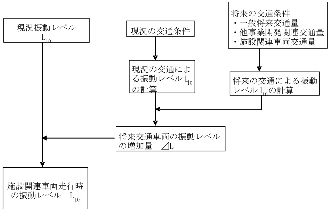
図 7-2-3-6 施設関連車両の走行に係る道路交通振動の予測手順
