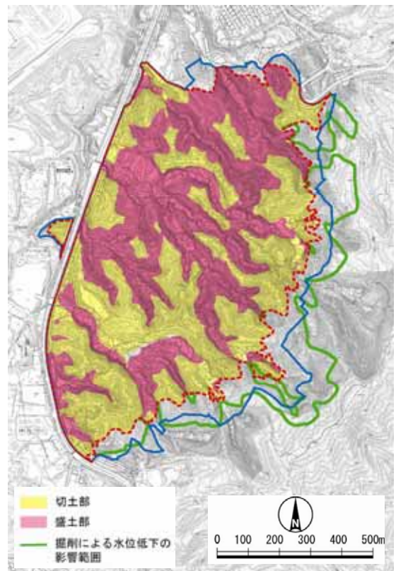
図 5 切土による流出影響範囲図
