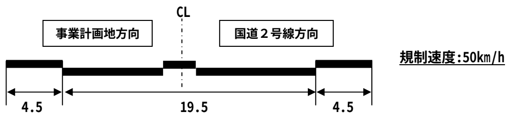
図 7-1-11(4) 道路条件(地点 D)
