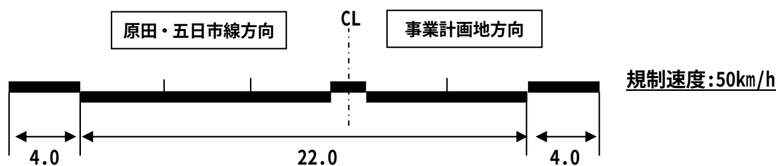
図 7-1-11(2) 道路条件(地点 B)
