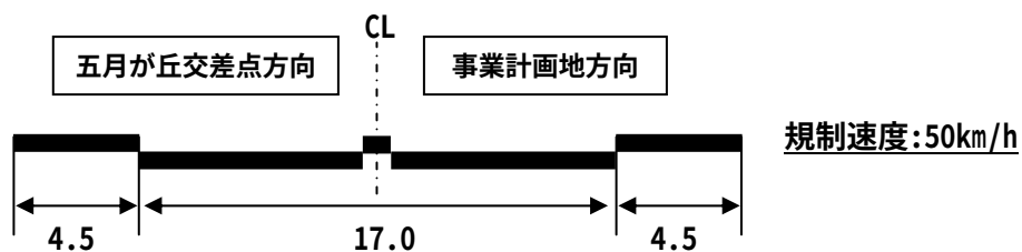
図 7-1-11(1) 道路条件(地点 A)
