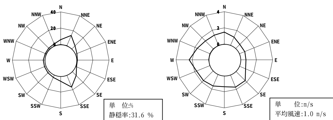
図 7-1-7(5) 風配図(左図)及び風向別平均風速(右図) (年間)
