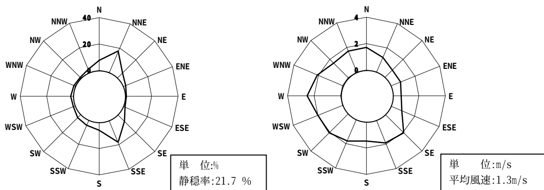
図 7-1-7(3) 風配図(左図)及び風向別平均風速(右図) (春季:平成 21 年 3 月 1 日～5 月 31 日)
