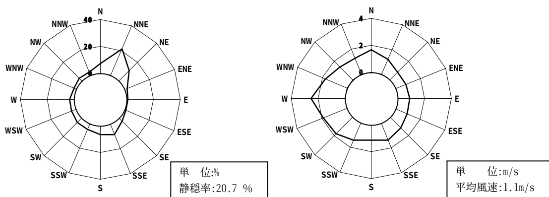
図 7-1-7(2) 風配図(左図)及び風向別平均風速(右図) (冬季:平成 20 年 12 月 1 日～平成 21 年 2 月 28 日)
