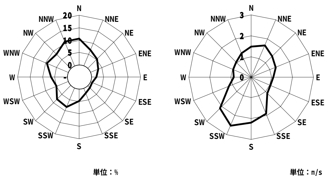
図7-1-4 風配図(左図)及び風向別平均風速(右図) (伴小学校測定局、平成21年度)
