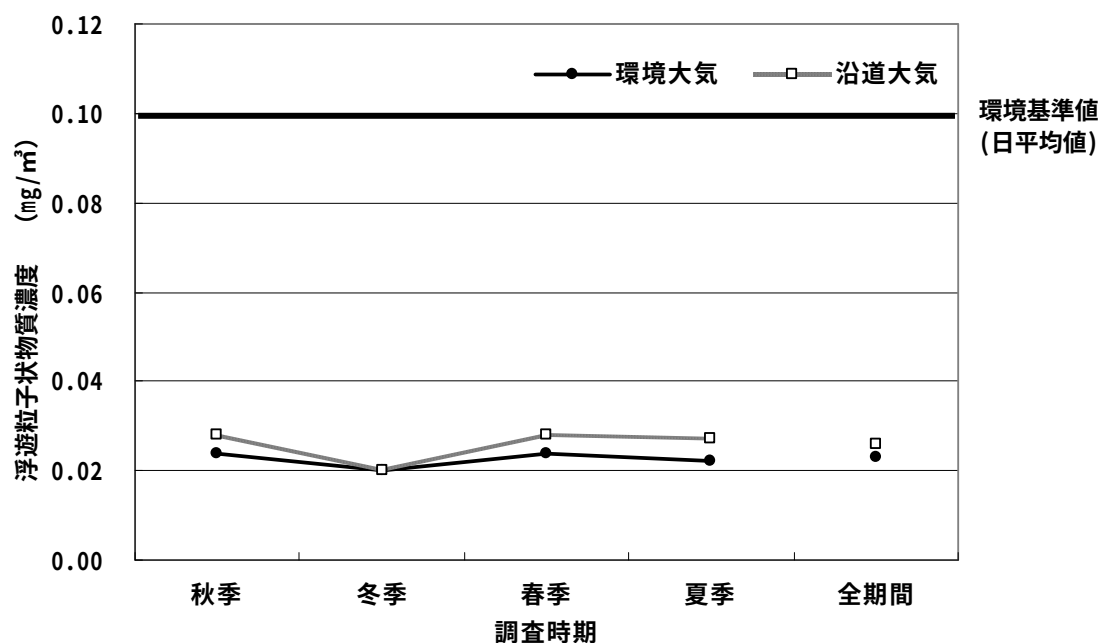
図 7-1-6 現地調査結果(浮遊粒子状物質、期間平均値)
