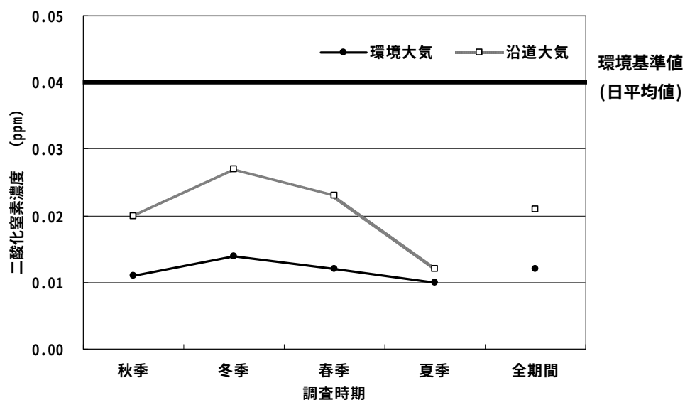
図 7-1-5 現地調査結果(二酸化窒素、期間平均値)
