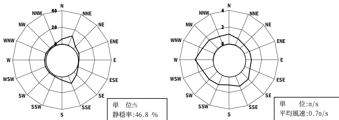
図 7-1-7(1) 風配図(左図)及び風向別平均風速(右図) (秋季:平成 20 年 9 月 1 日～11 月 30 日)
