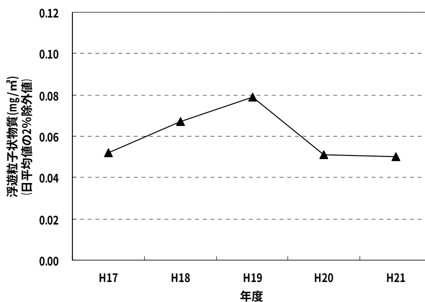
図 7-1-2(2) 浮遊粒子状物質の年間 2%除外値の経年変化 (伴小学校測定局)
