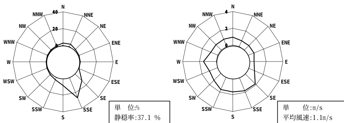
図 7-1-7(4) 風配図(左図)及び風向別平均風速(右図) (夏季:平成 21 年 6 月 1 日～8 月 31 日)
