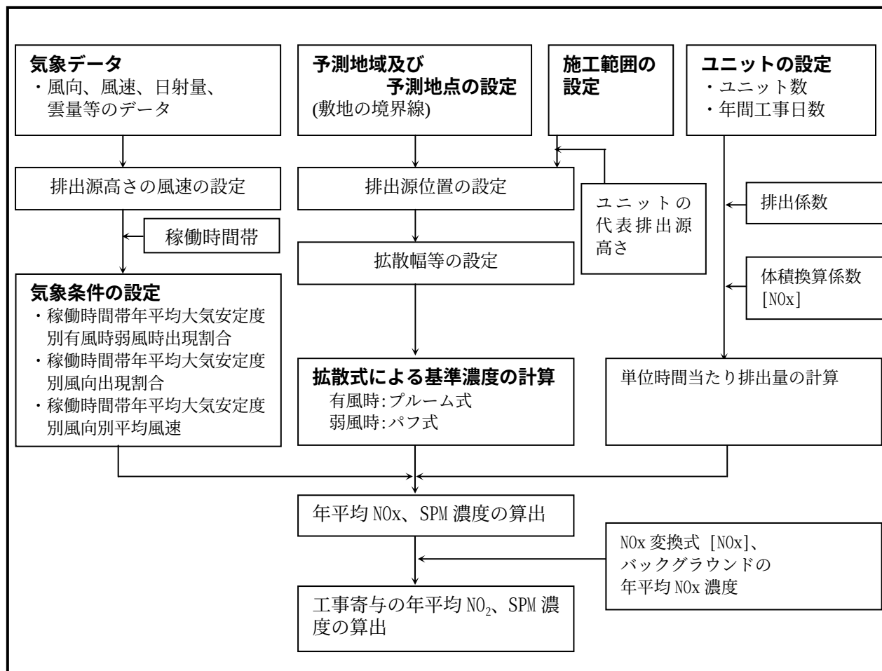
図 7-1-12 予測フロー(建設機械の稼働による大気質の変化)
