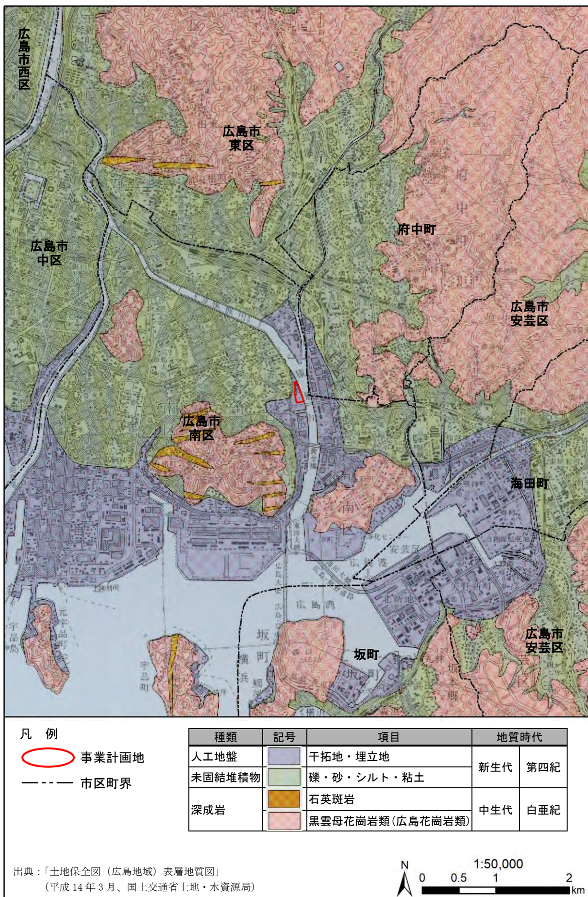
図 3-12 事業計画地及びその周辺の表層地質図
