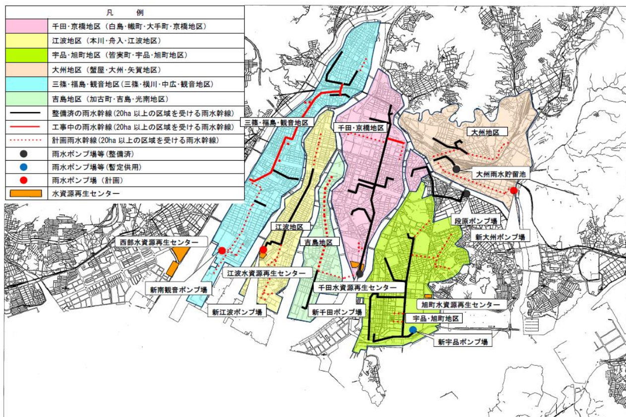
下水道浸水対策事業の整備状況（令和5年度末）
