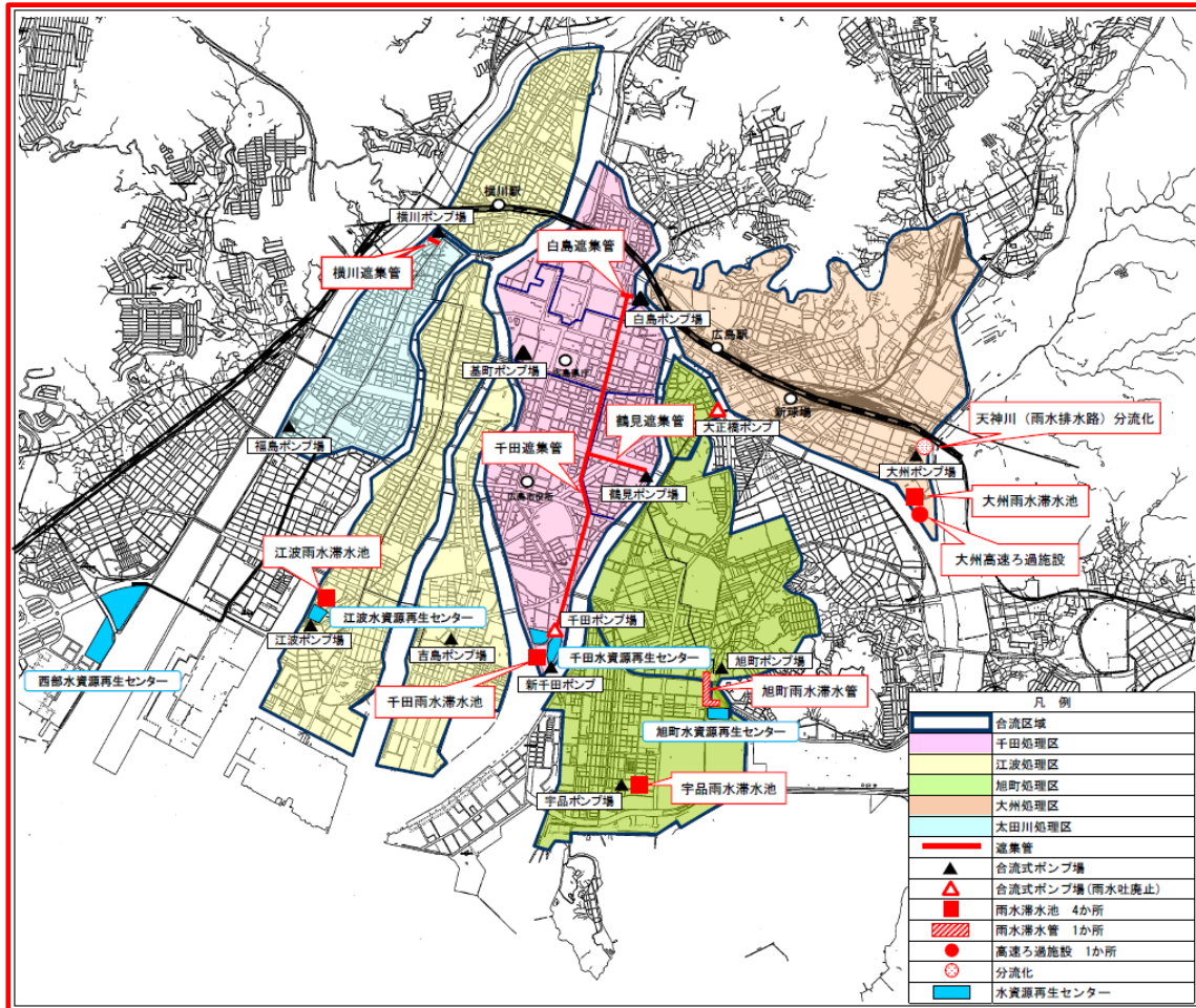
合流式下水道改善状況図（令和6年4月1日現在）
