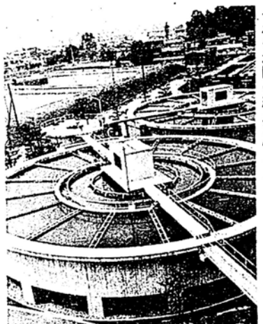
水源地内の強制沈デソ池
