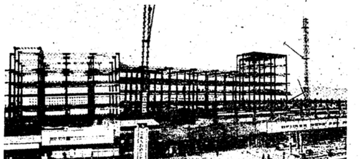
鉄骨の組立てをほとんど終った民衆駅の建設工事
