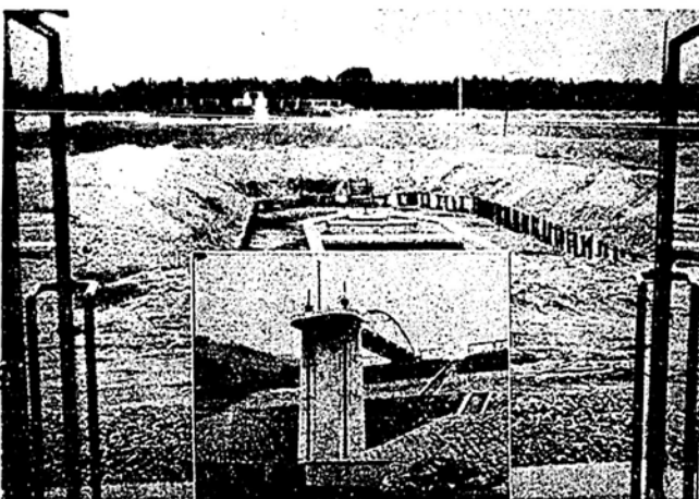
人口の増加に伴い取水量を増すために新しく建設されたのがこの戸坂取水場で(中央は取入口)ここから管で牛田浄水場に送られ、飲料水になります。
