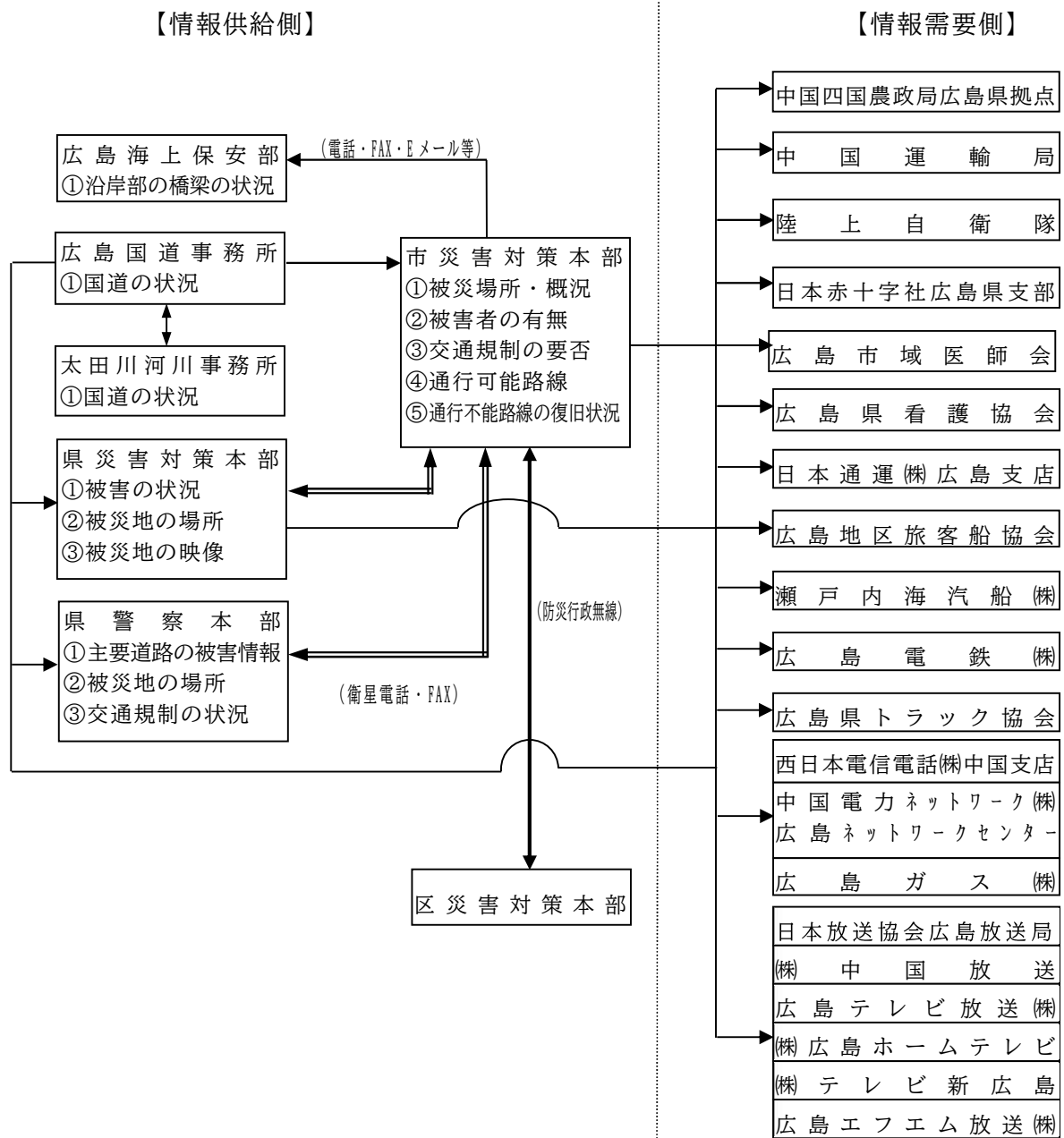
図3-3-8 道路・橋梁情報体系
