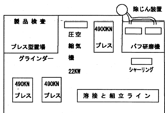
機械施設の配置図
