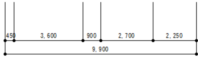
第19号棟 1120号室(3Kタイプ 41.85 m 2 )
