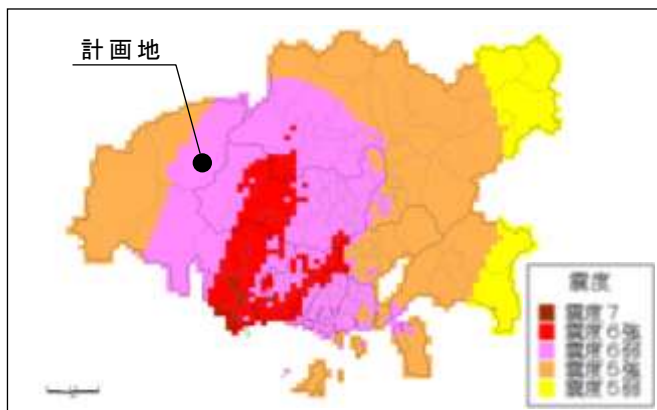
図 震度分布（五日市断層による地震）
