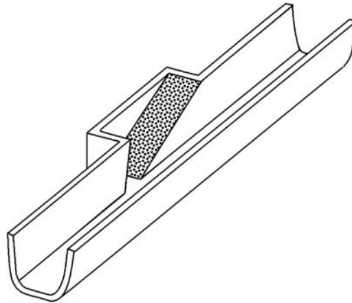
図 7-10-40 小型動物脱出対応型の水路のイメージ図
