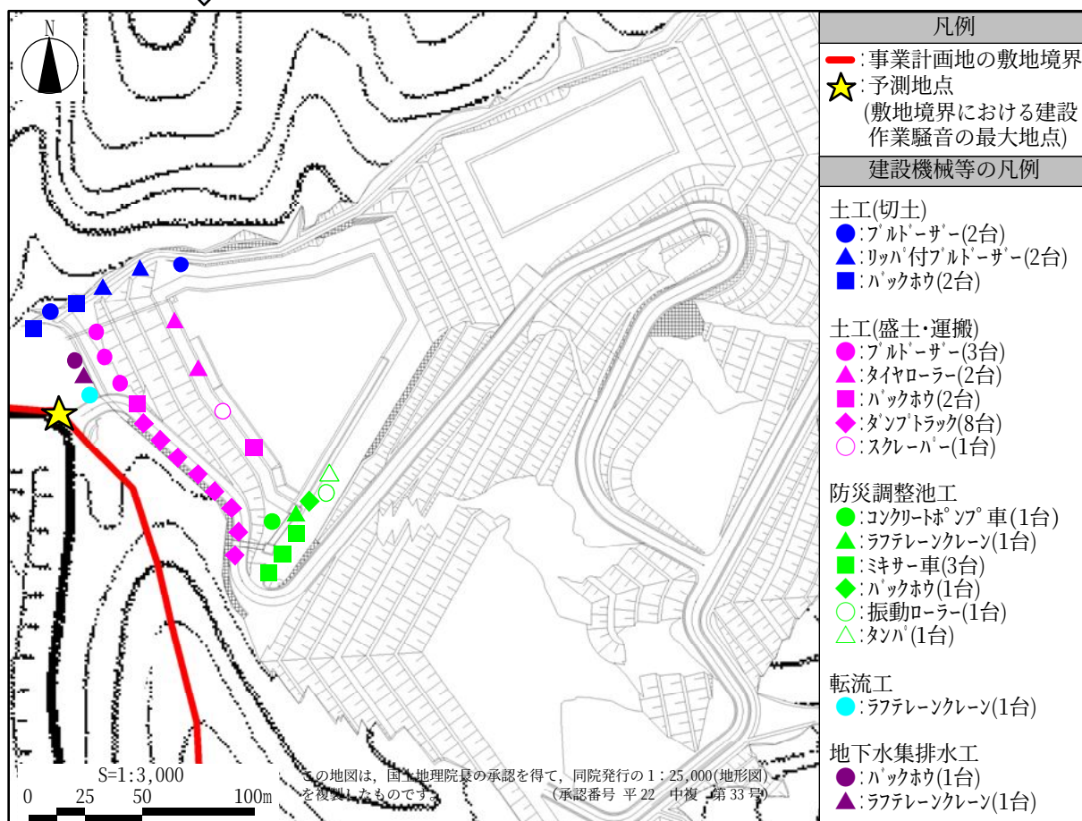
図7-2-8(1) 予測地点及び建設機械の稼働位置図(ケース1)
