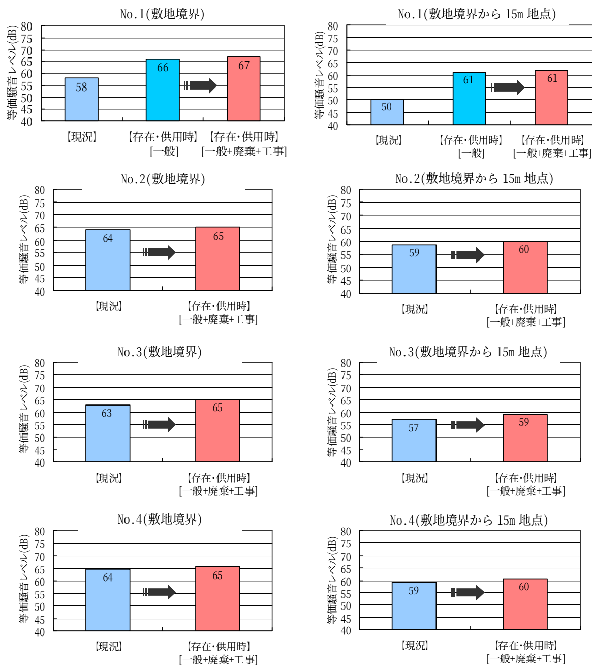
図 7-2-21 現況及び予測結果
