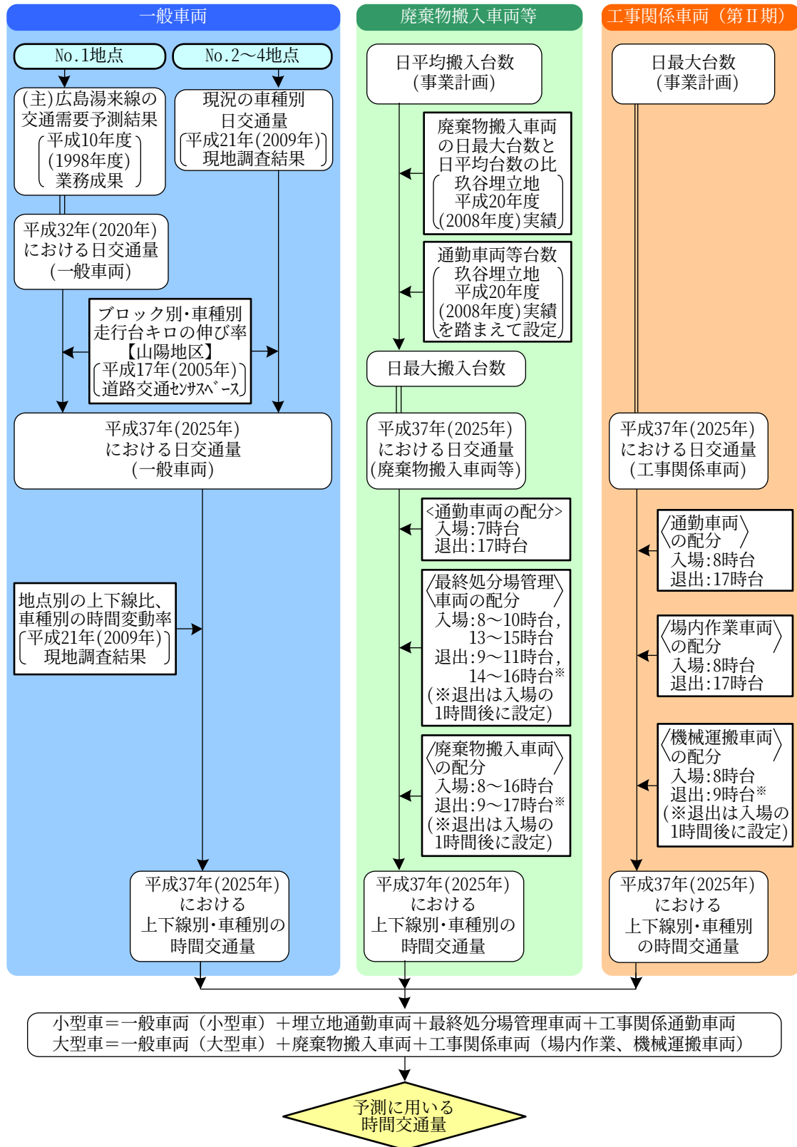
図 7-2-19 将来交通量の設定方法
