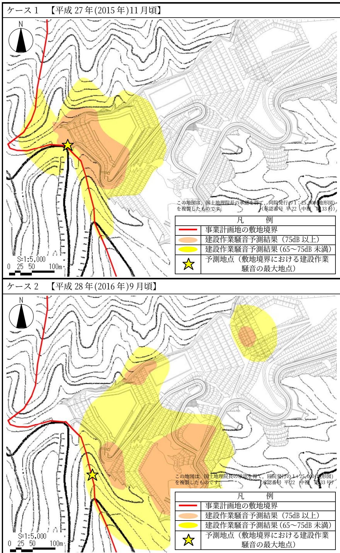
図 7-2-9 建設作業騒音予測結果
