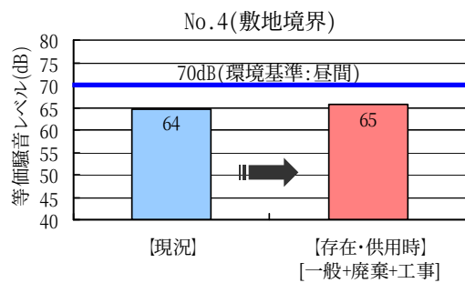
図 7-2-22 評価結果（存在・供用時の道路交通騒音）
