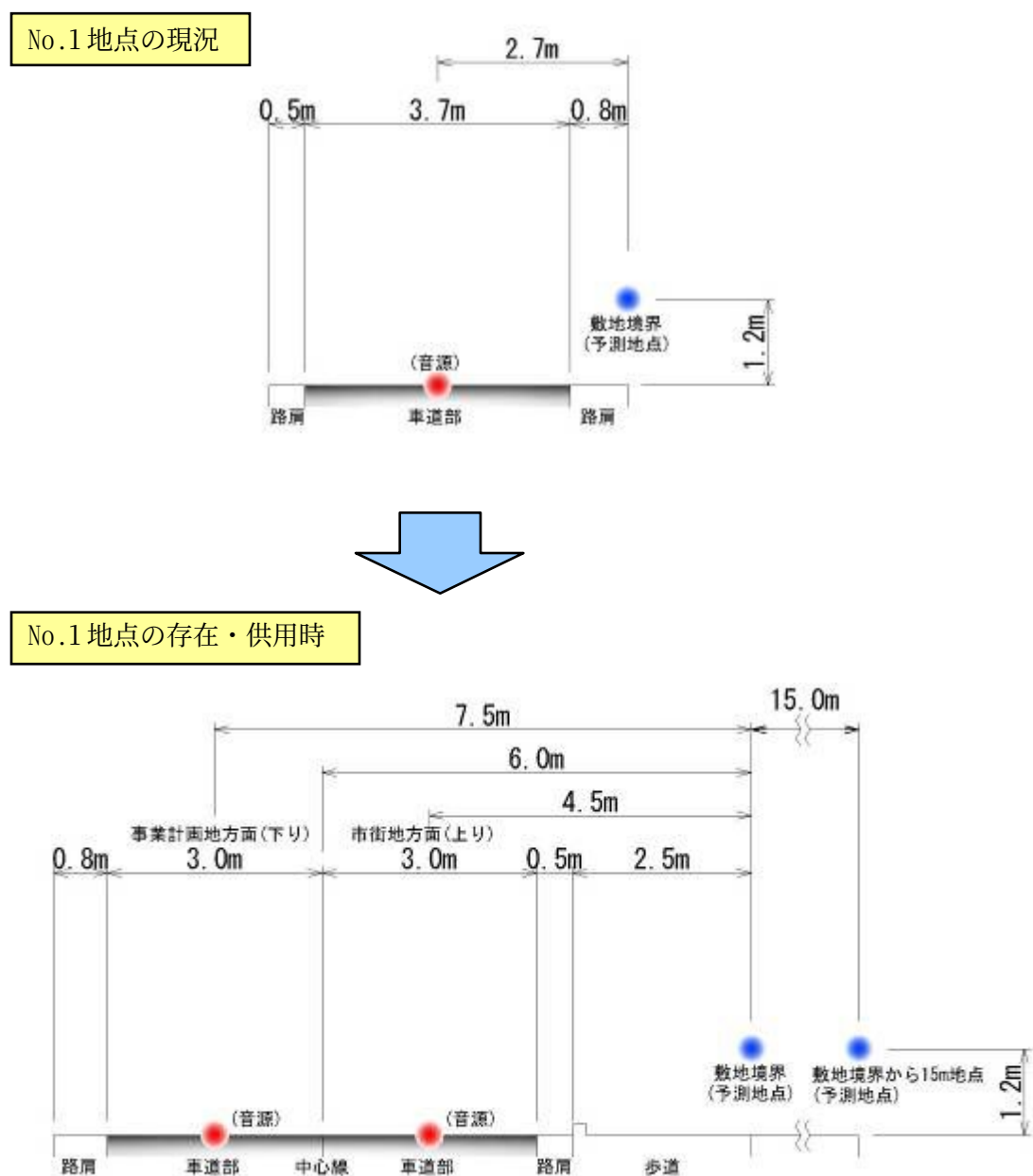
図7-2-18 予測地点（現況及び存在・供用時の道路構造 No.1）
