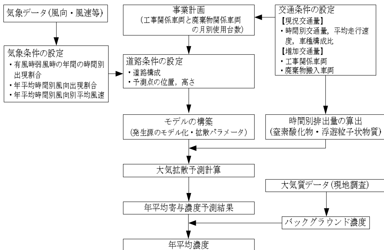
図 7-1-31 予測フロー
