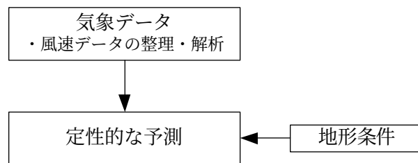
図 7-1-19 予測フロー
