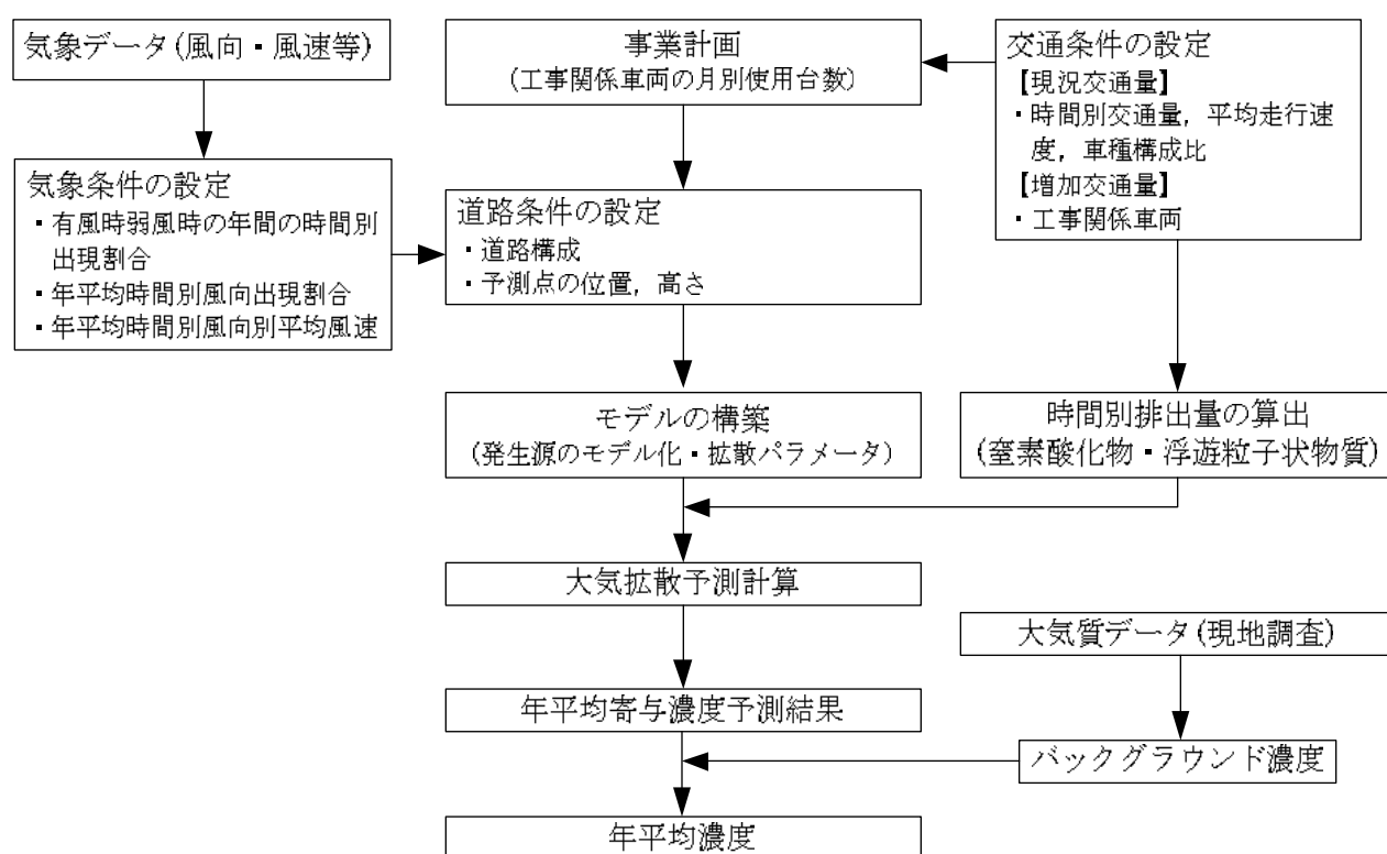
図 7-1-21 予測フロー
