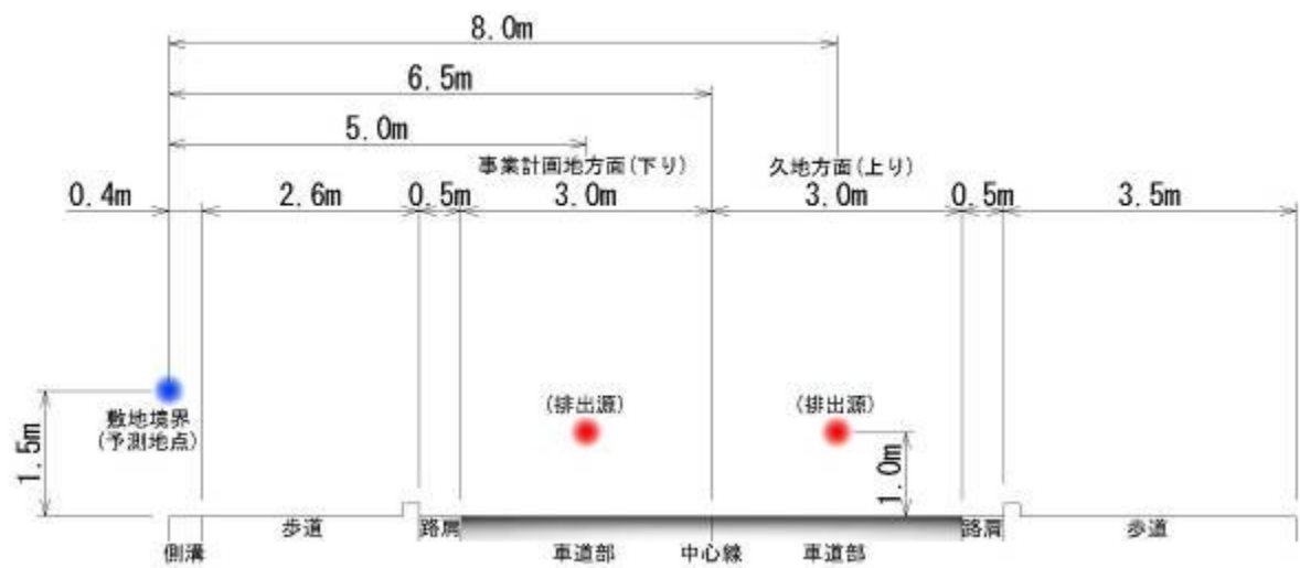
断面図(S=1/100)
