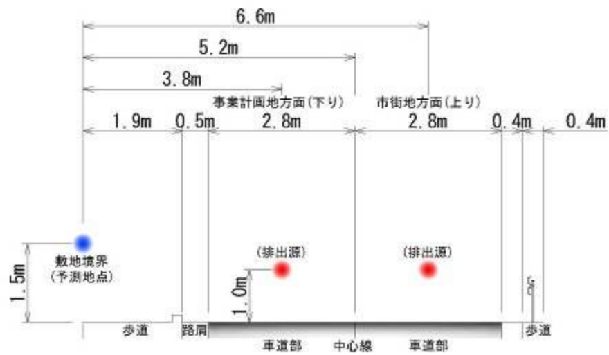
断面図 (S=1/100)
