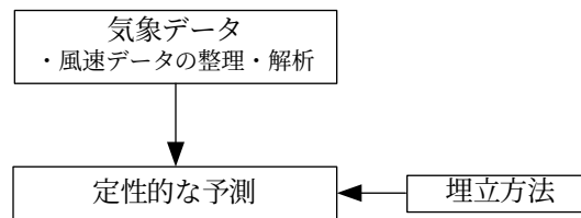
図 7-1-29 予測フロー
